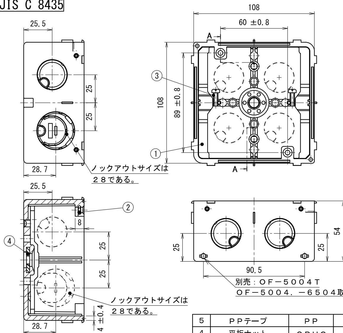
A-A 断面図
